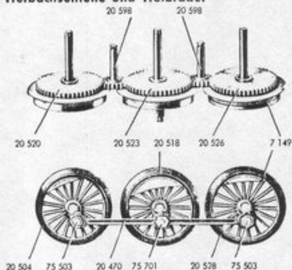
Fig. 6 Gestänge
