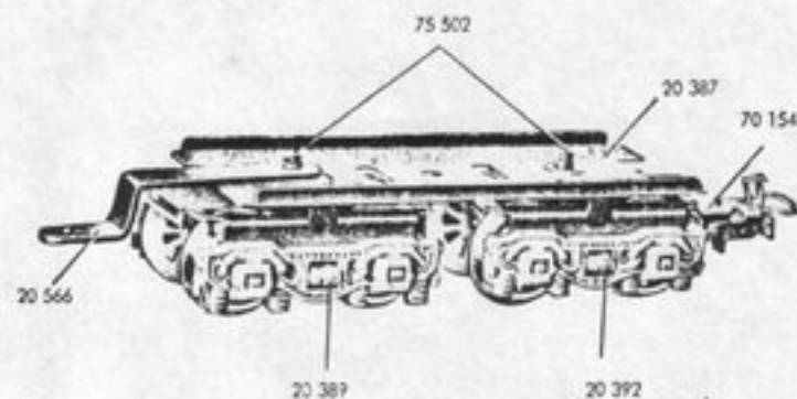
Fig. 2 Fahrgestell
