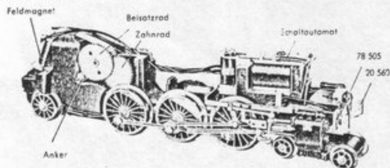
Fig. 2 Fahrgestell (Getriebeseite aufgeschnitten)
