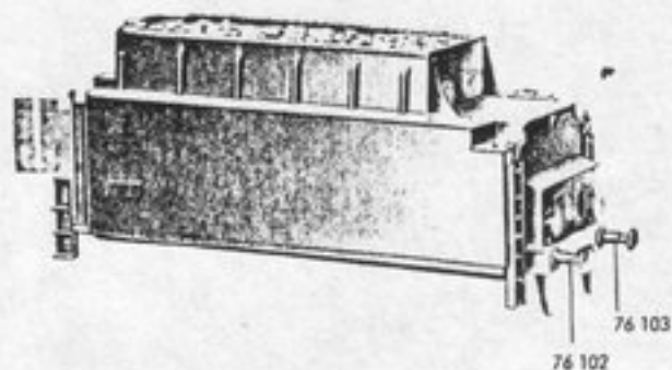
Fig. 2 Fahrgestell
